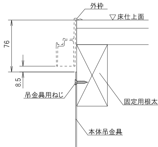
本体吊金具まわり断面
